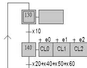
GRAFCET N°4 (Allumer "leds" aux étages)
