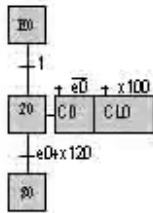
MACRO ETAPE M0 (vue étape 0)
