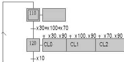
GRAFCET N°2 (Clignotement des "leds")
