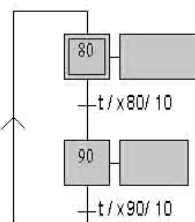
GRAFCET N°3 (base de temps)
