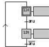
GRAFCET auxiliaire (Amplitude tension)
