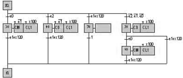
MACRO ETAPE M1 (vue étape 1)
