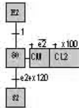
MACRO ETAPE M2 (vue étape 2)
