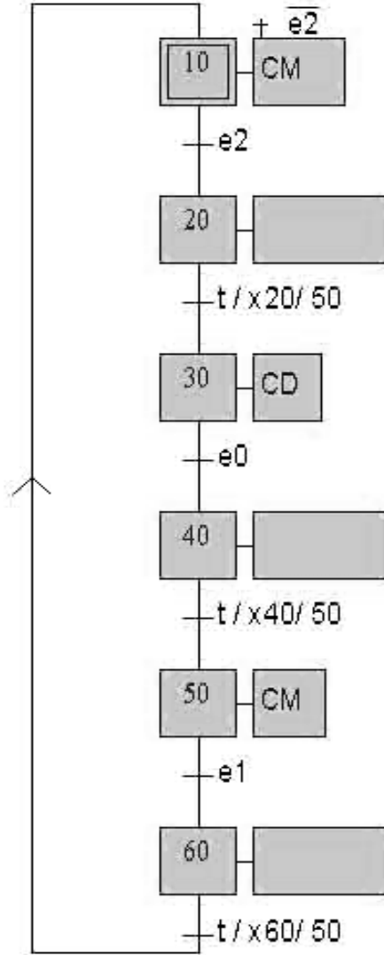
GRAFCET N°2
