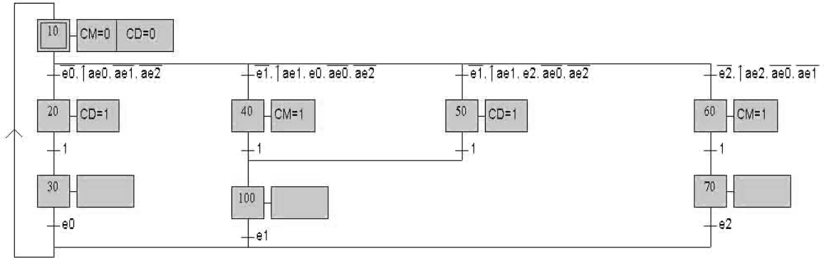
GRAFCET N°1 (Gestion montée/descente)
