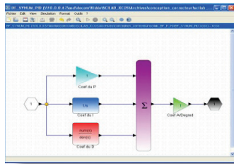
Corrector PID editado bajo Xcos Código generado por D_Scil
