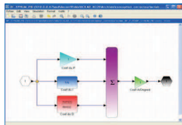
Correcteur PID édité sous Xcos
